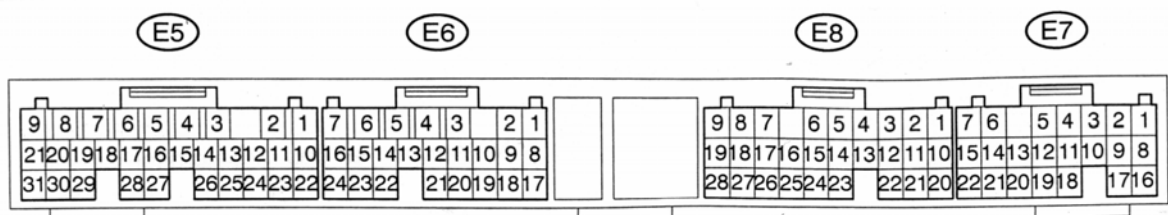
Bornes de l'ECU (vue de face)
