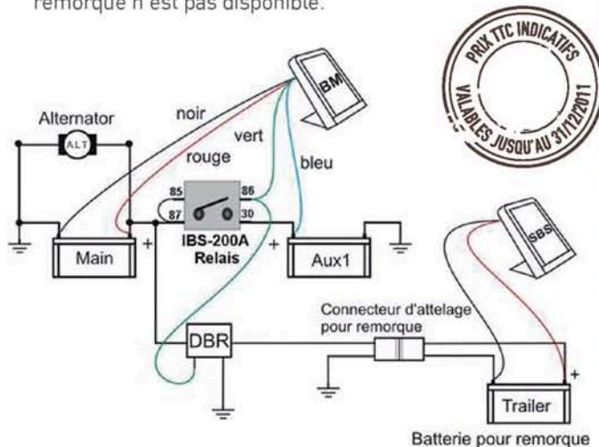
Batterie pour remorque Exemple du montage
