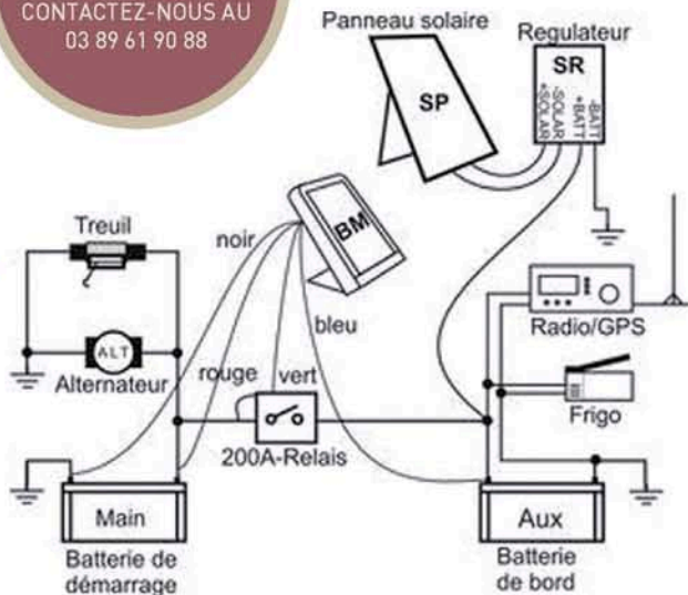
Monitor d'un Dual Batterie Système monté dans un véhicule
